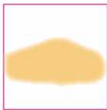
せっかいせき 石灰石
